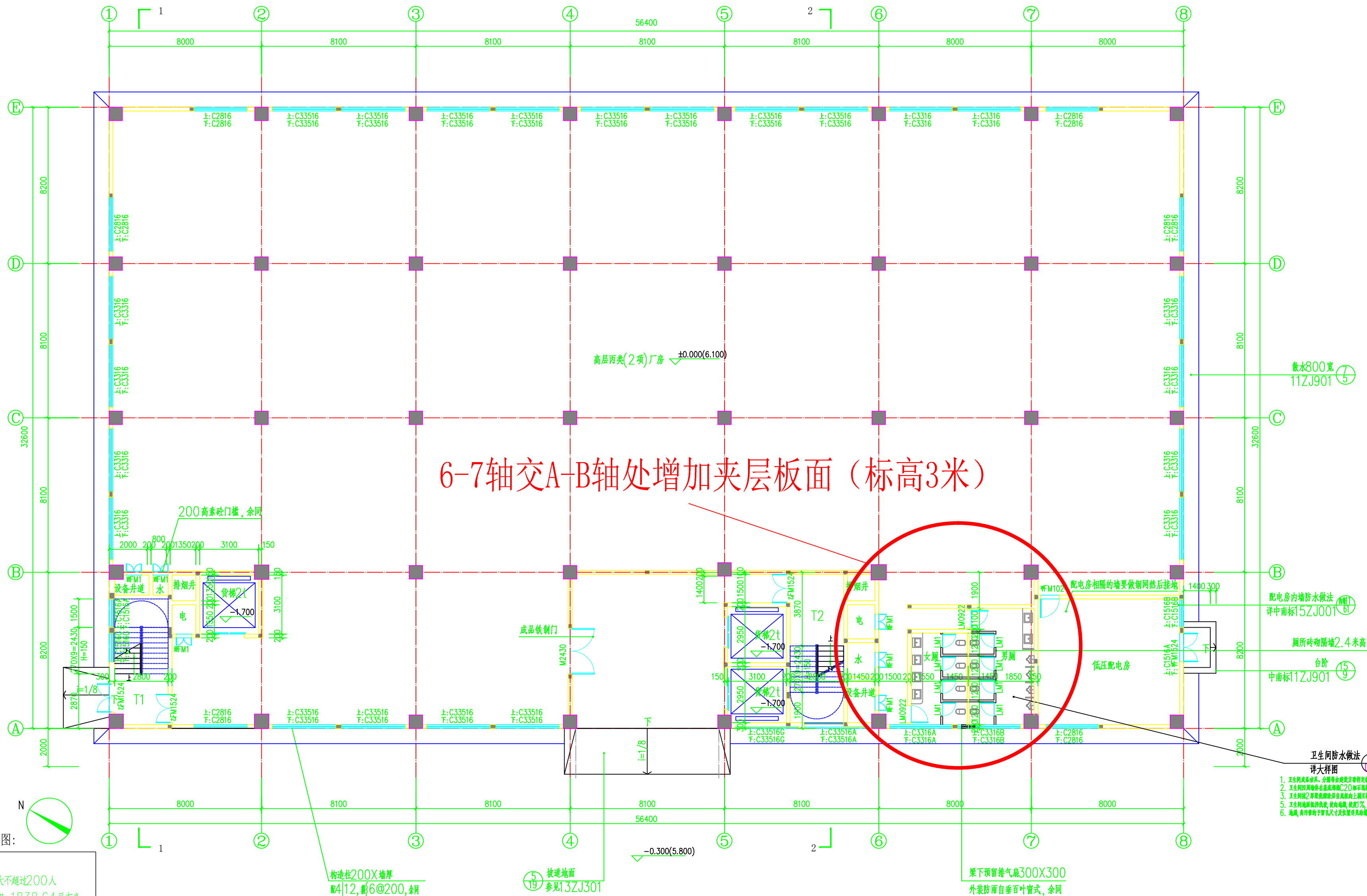
厂房首层平面 1:100
