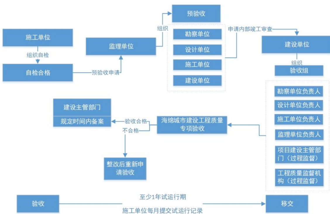
图 C 海绵城市建设工程验收程序流程图
