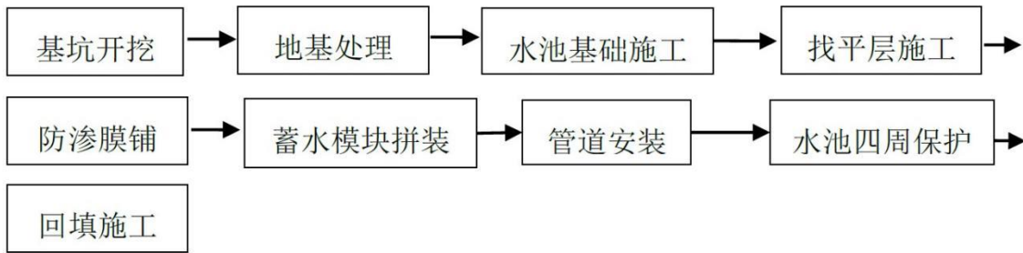
图 7-2 蓄水模块水池施工工序
