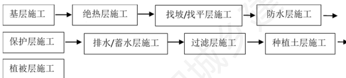
图 6-2 绿色屋顶施工工序
