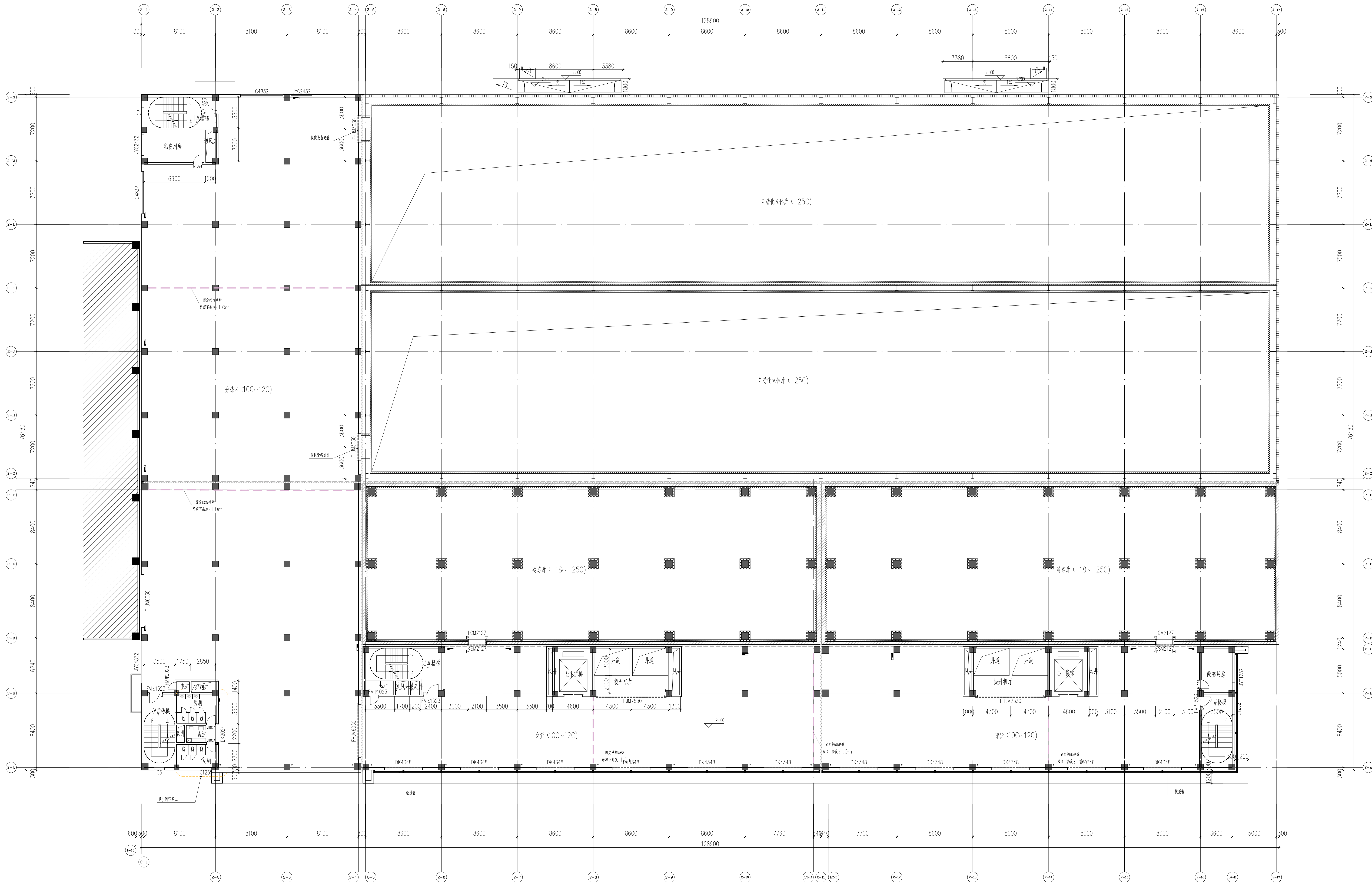
二层平面图 1:150
