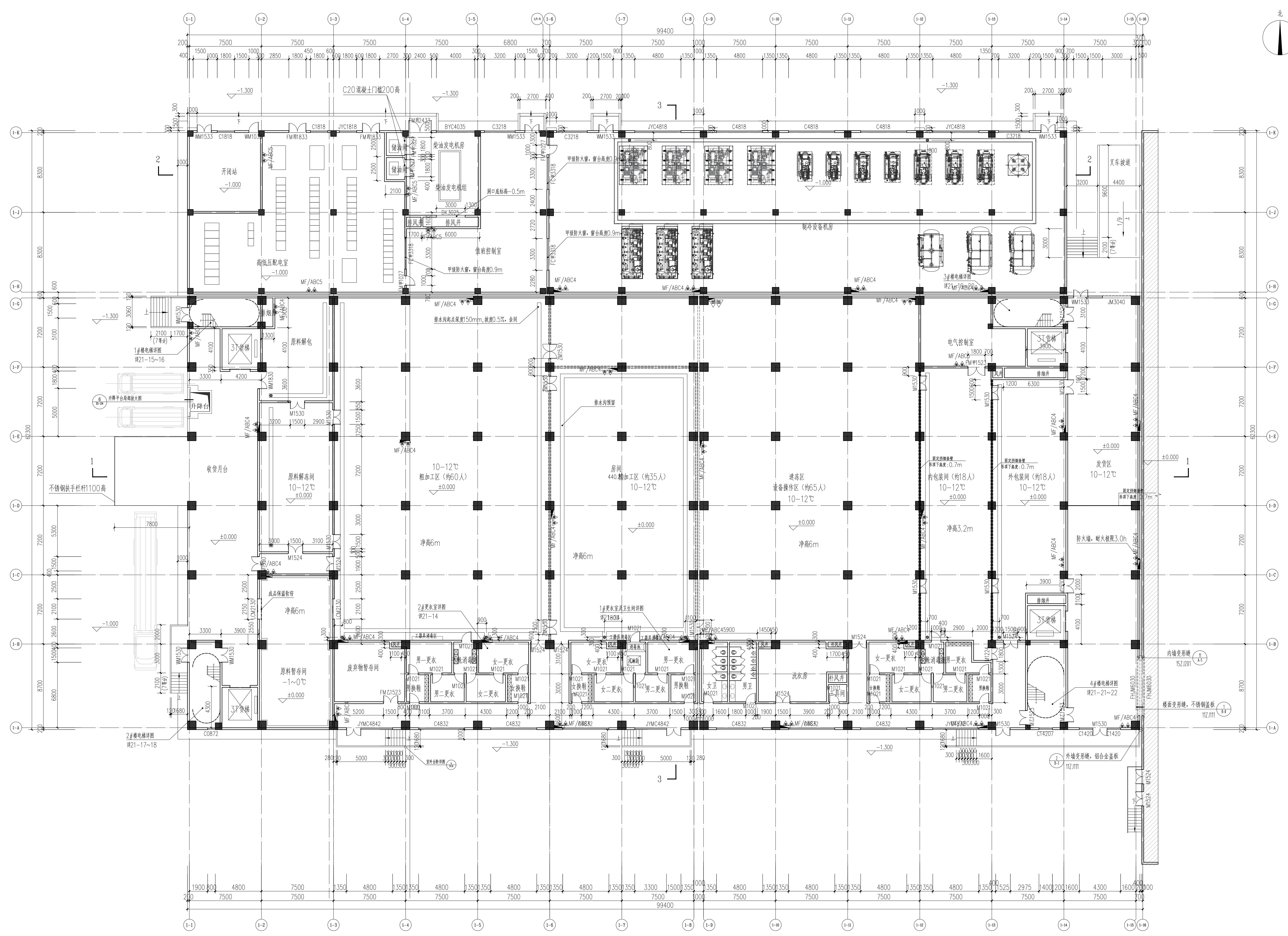
一层平面图 1:150
