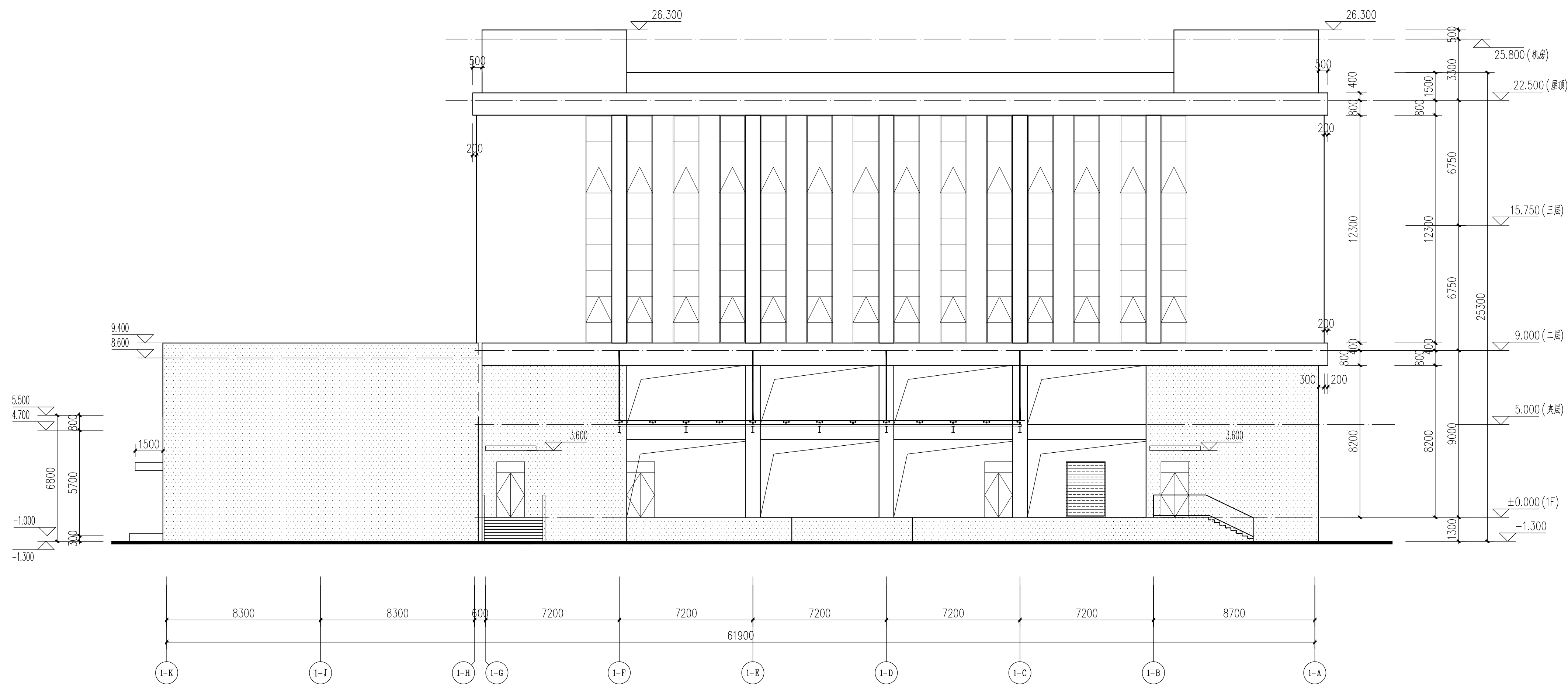
14~15立面图 1:150
