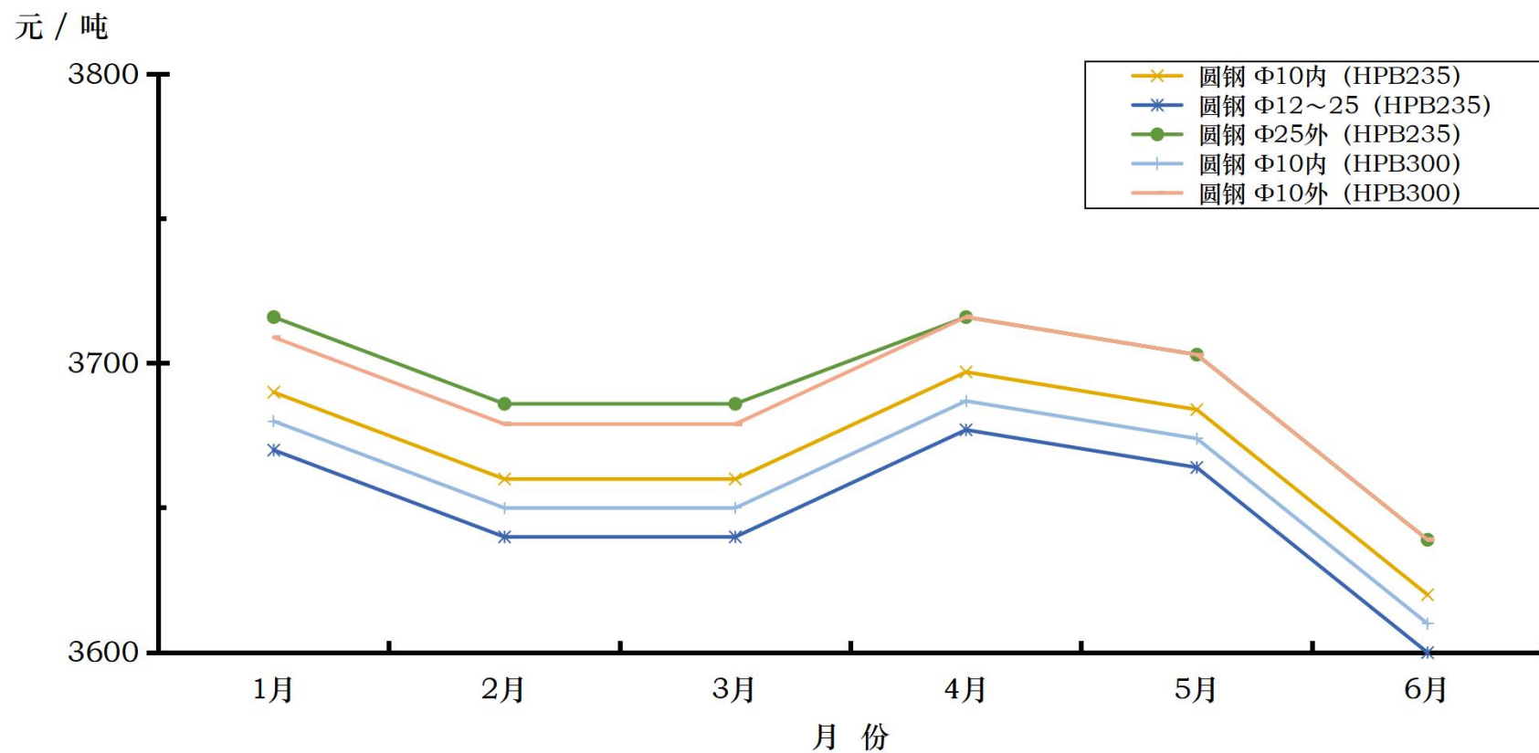
2026年上半年圆钢价格走势图
