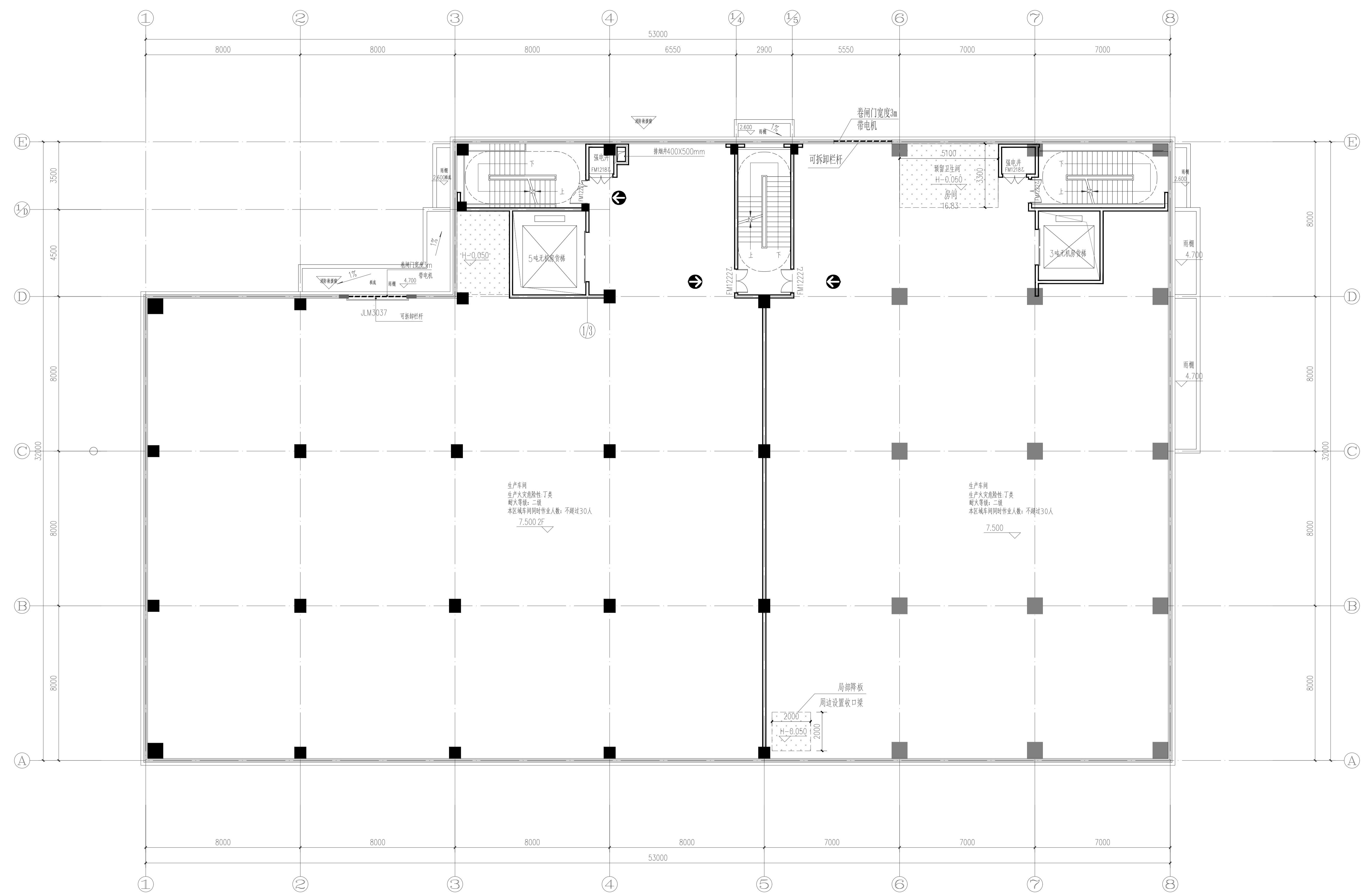
二层平面图 1:100
