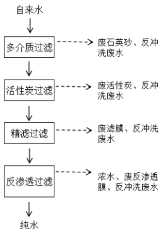
图2-3 纯水制备流程图
