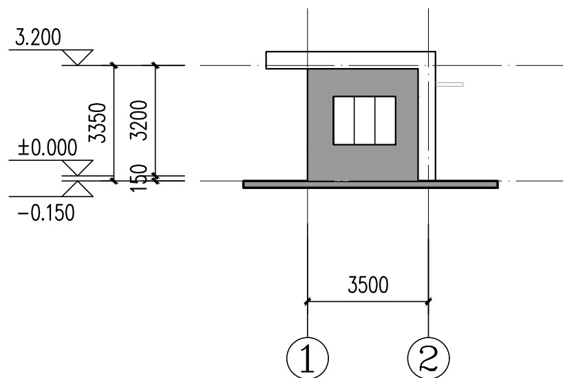
1-2轴立面图 1:150
