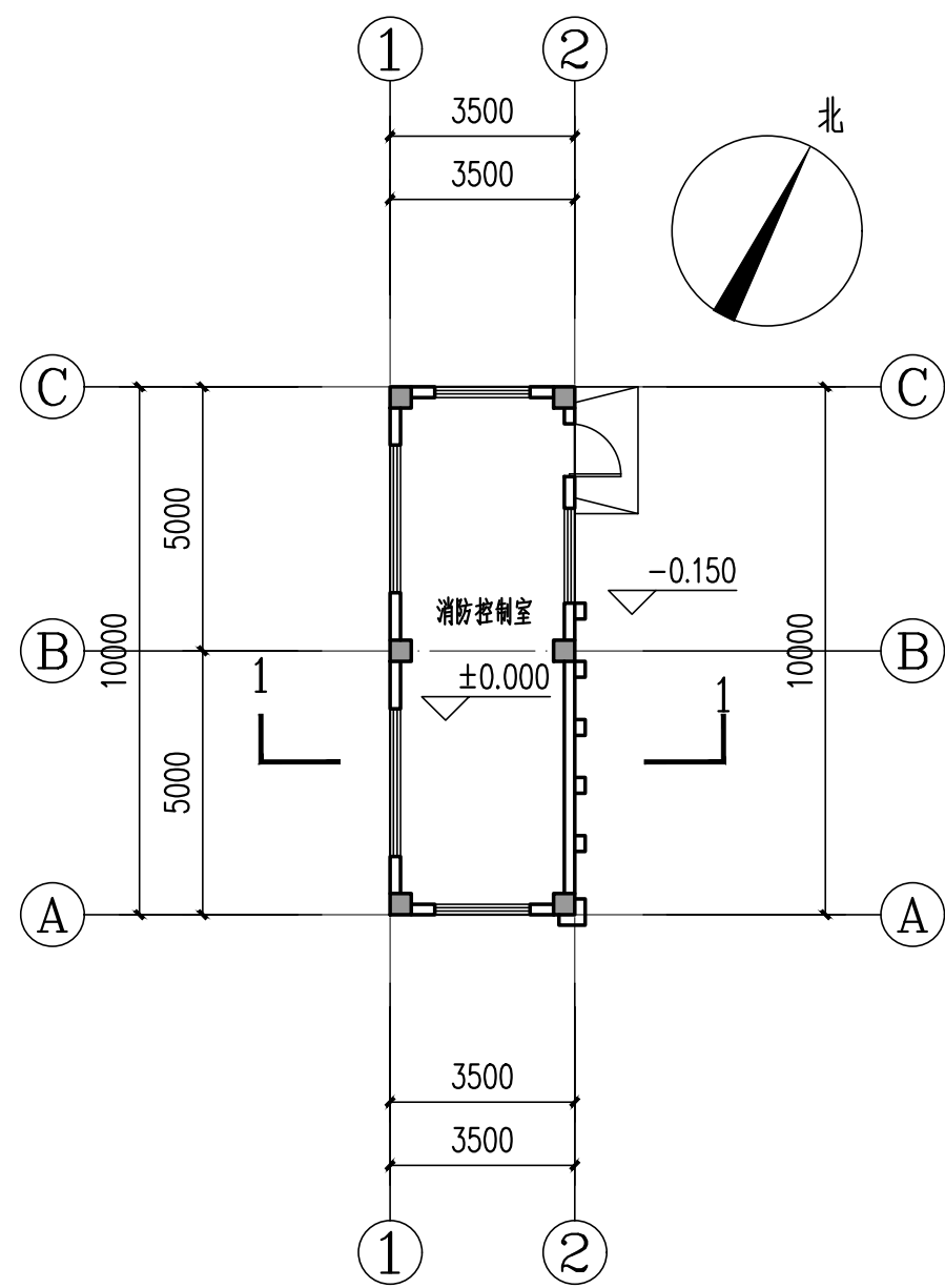
一层平面图 1:150
