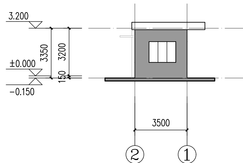
2-1轴立面图 1:150
