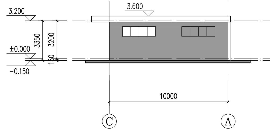
C-A轴立面图 1:150
