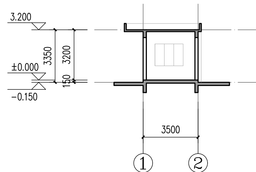
1-1剖面图 1:150
