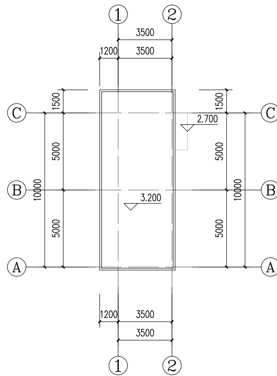
屋面层平面图 1:150
