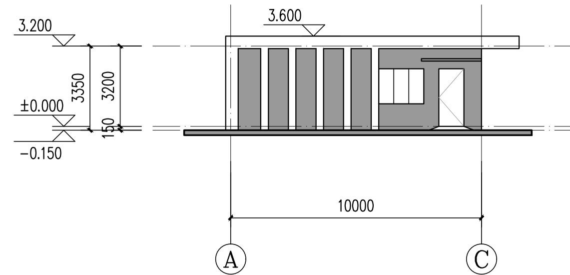
A-C轴立面图 1:150
