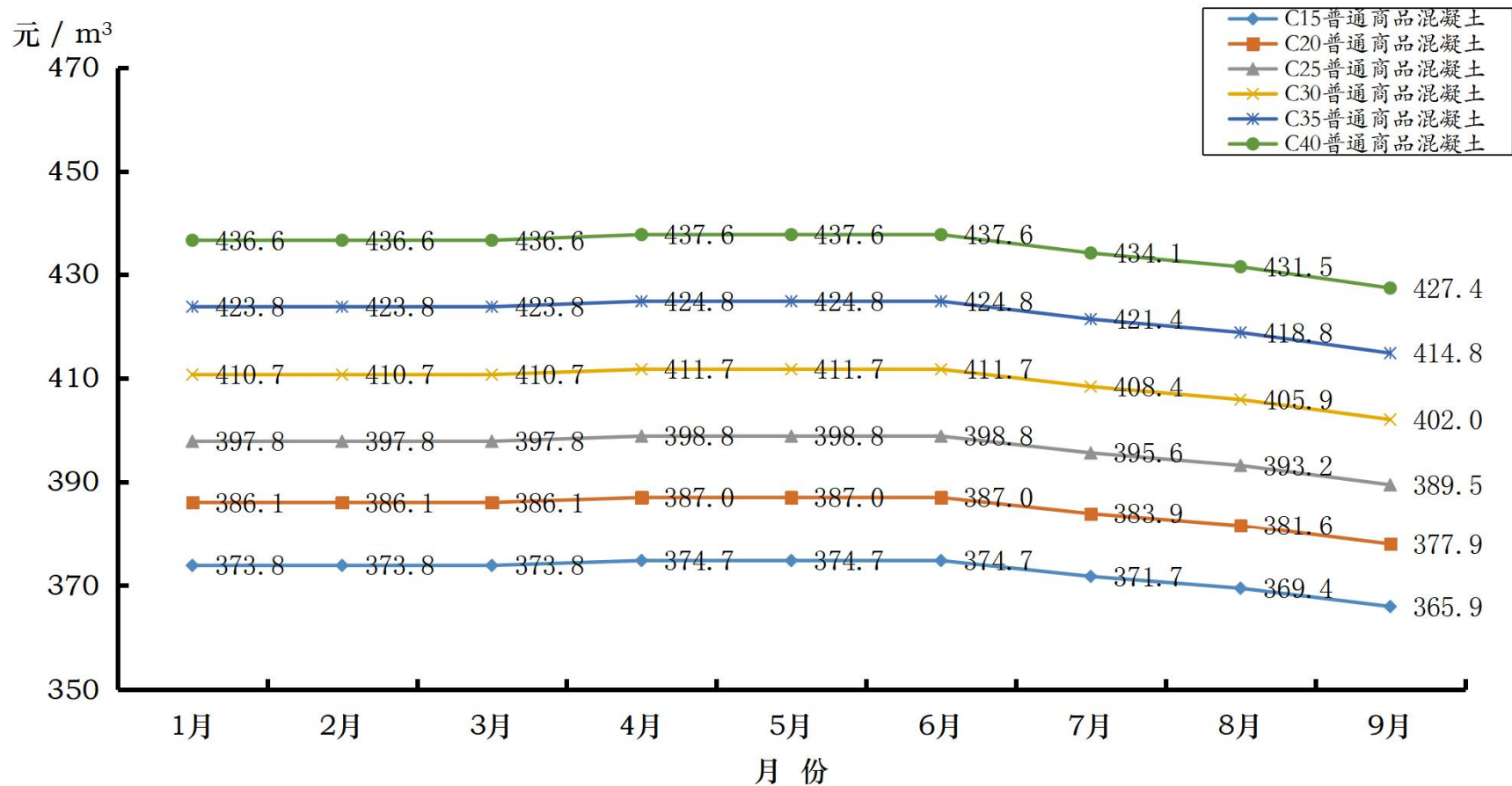
2025年前三季度商品混凝土价格走势
