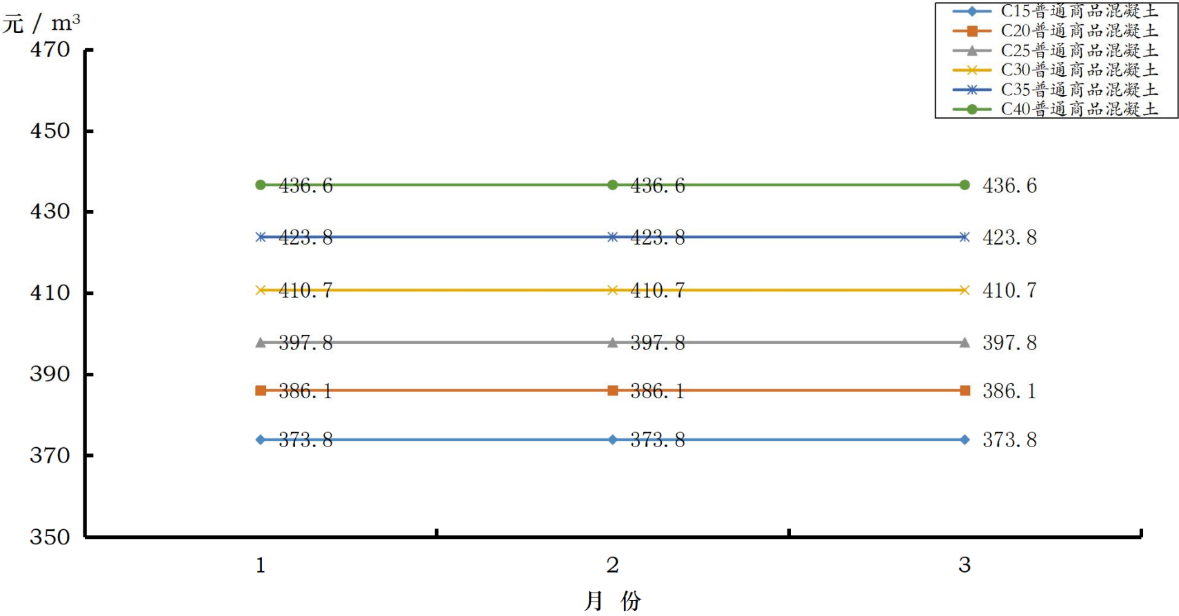
2025年第一季度商品混凝土价格走势
