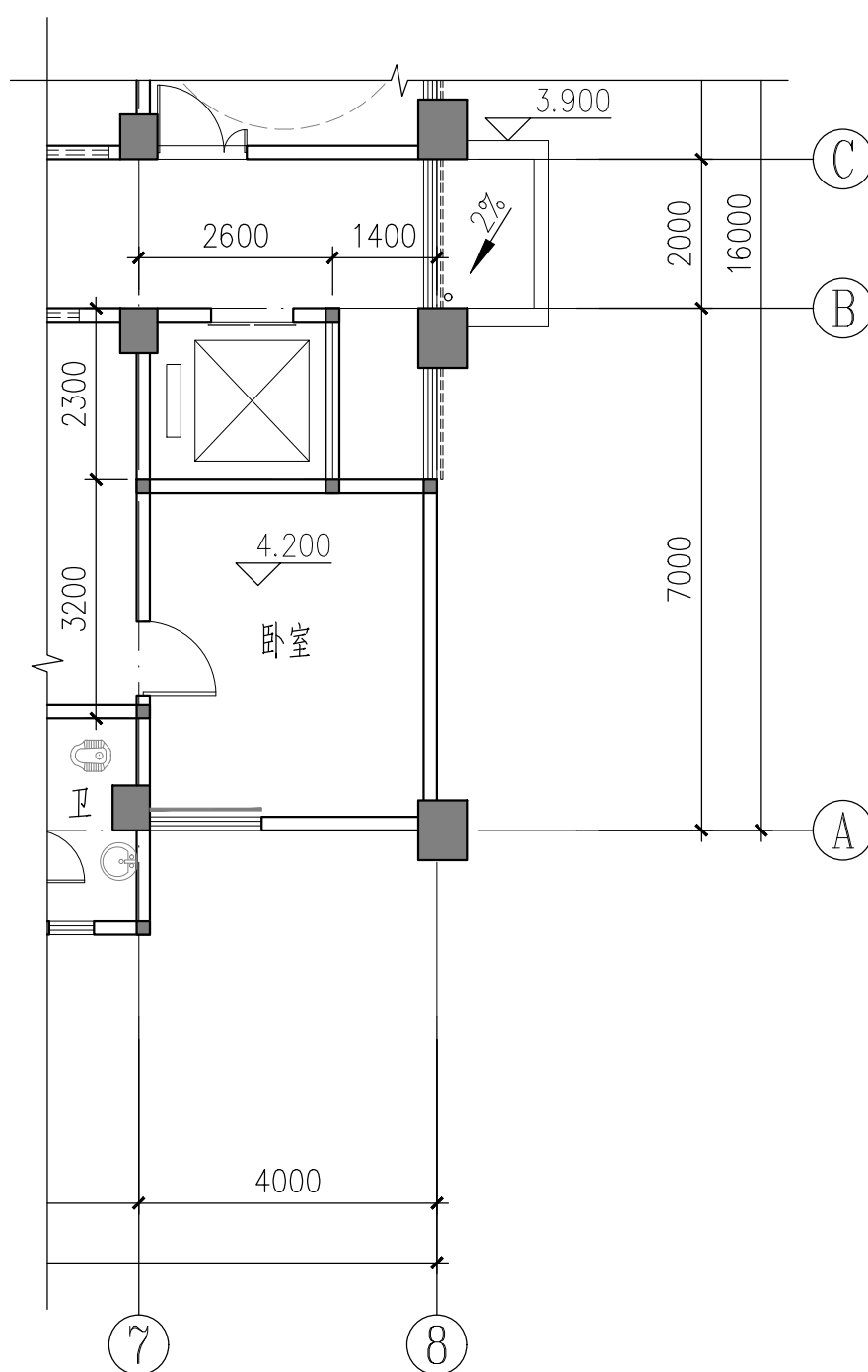
二层平面图 1:100
