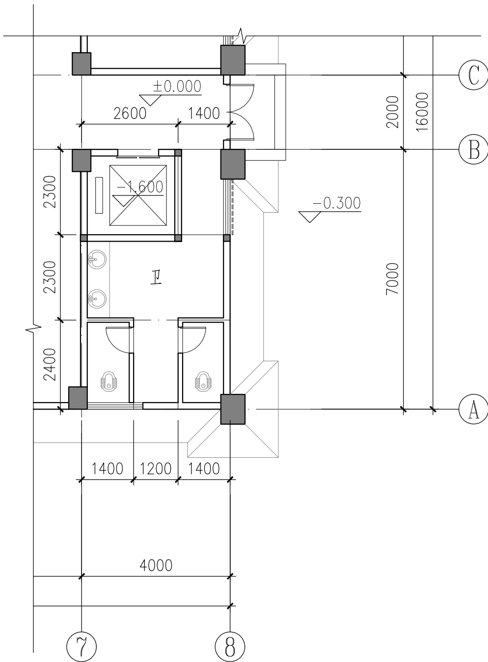
一层平面图 1:100
