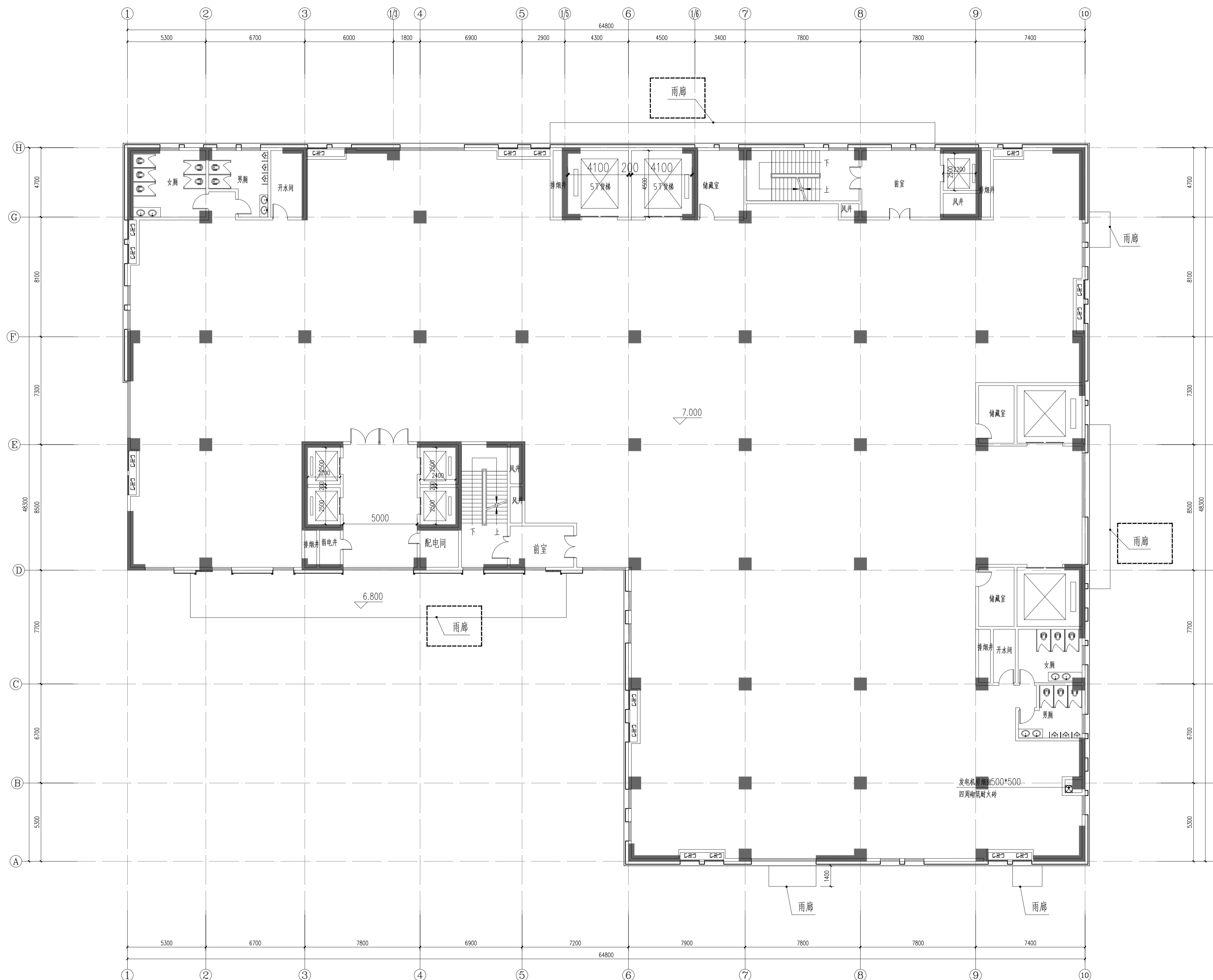
二层平面图 1:150
